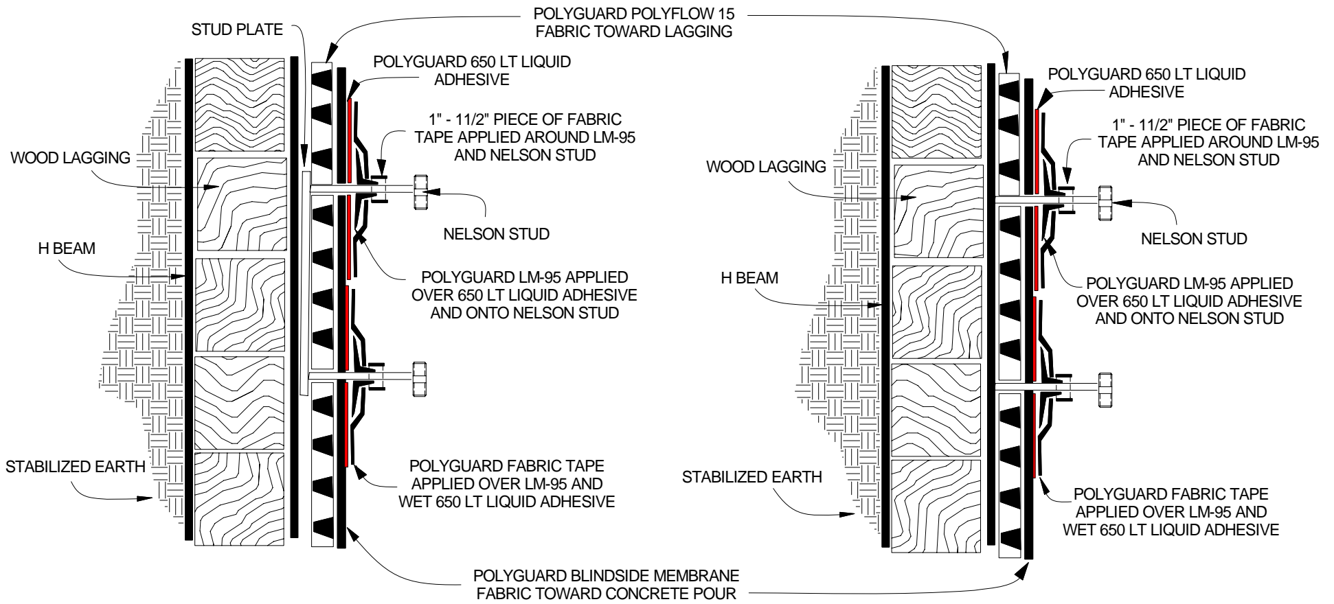
NELSON STUD WELDED TO STUD PLATE
